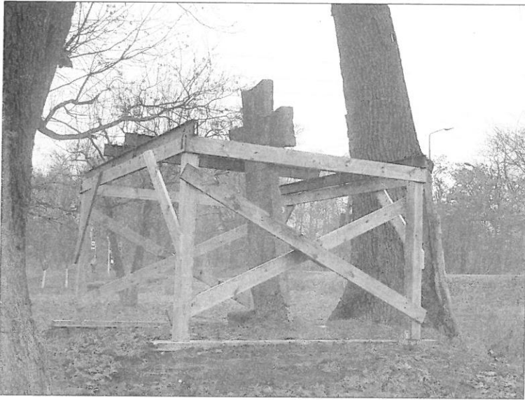
Ilustr. 3. Krzyż pokutny w Stargardzie. Stelaż zabezpieczający statykę obiektu podczas podnoszenia dźwigiem w trakcie prac konserwatorskich. Fot. A. Majewska – Muzeum w Stargardzie
